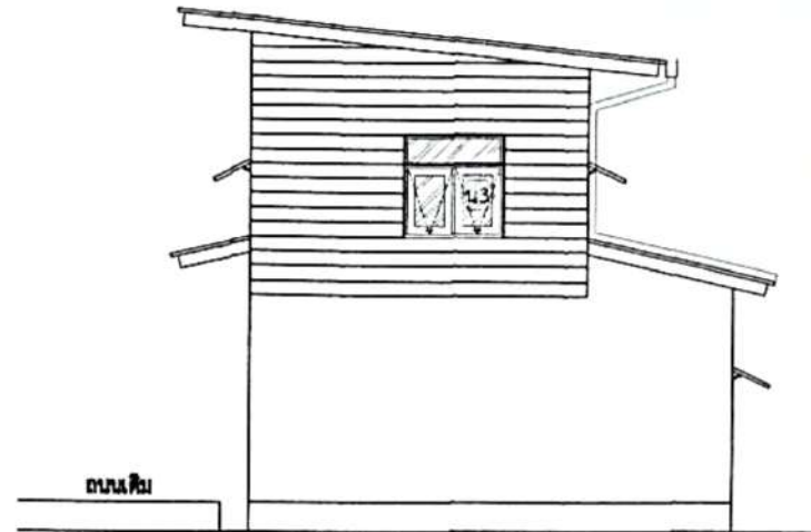
รูปด้าน ④ SCALE 1:100
