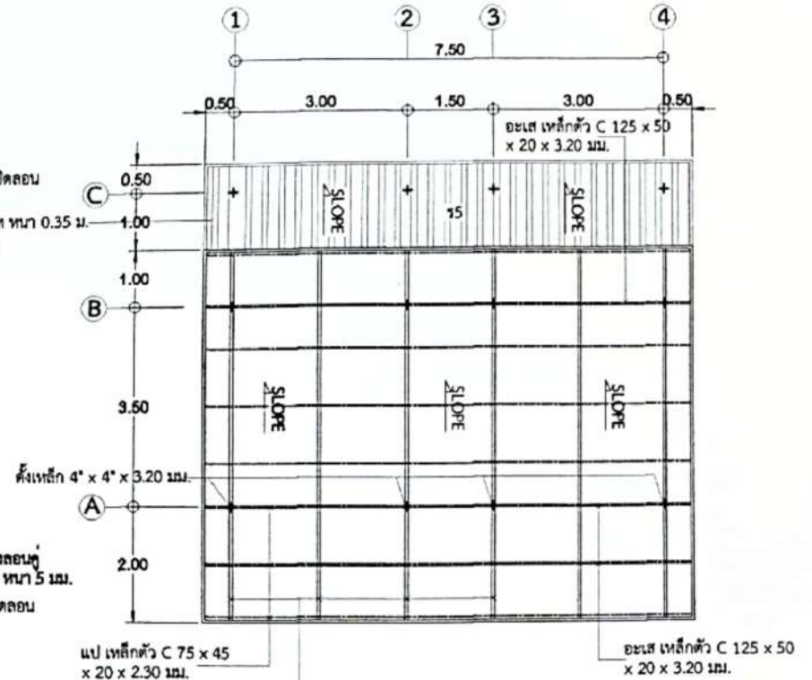
แบบโครงสร้างหลังคา SCALE 1:100
