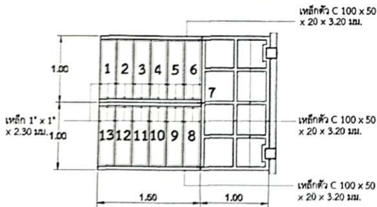
แบบขยายโครงเหล็กบันได SCALE 1:50
