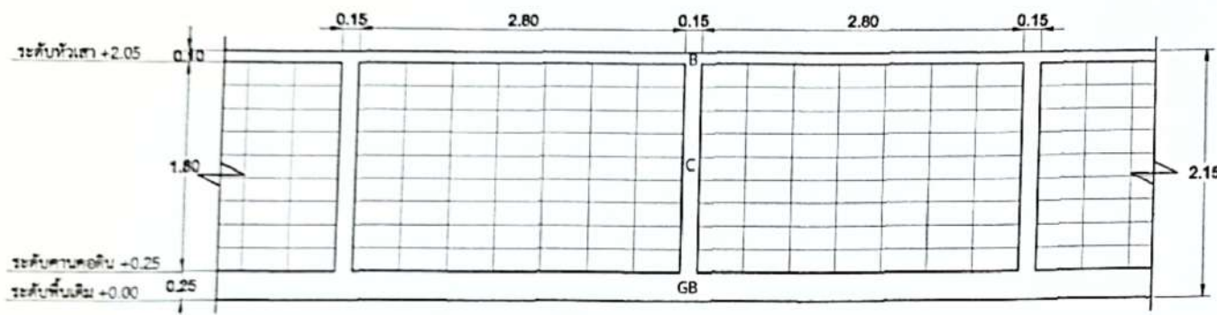
รูปด้าน SCALE 1:50
