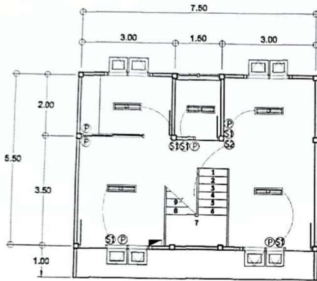
แบบไฟฟ้าชั้นล่าง SCALE 1:100
