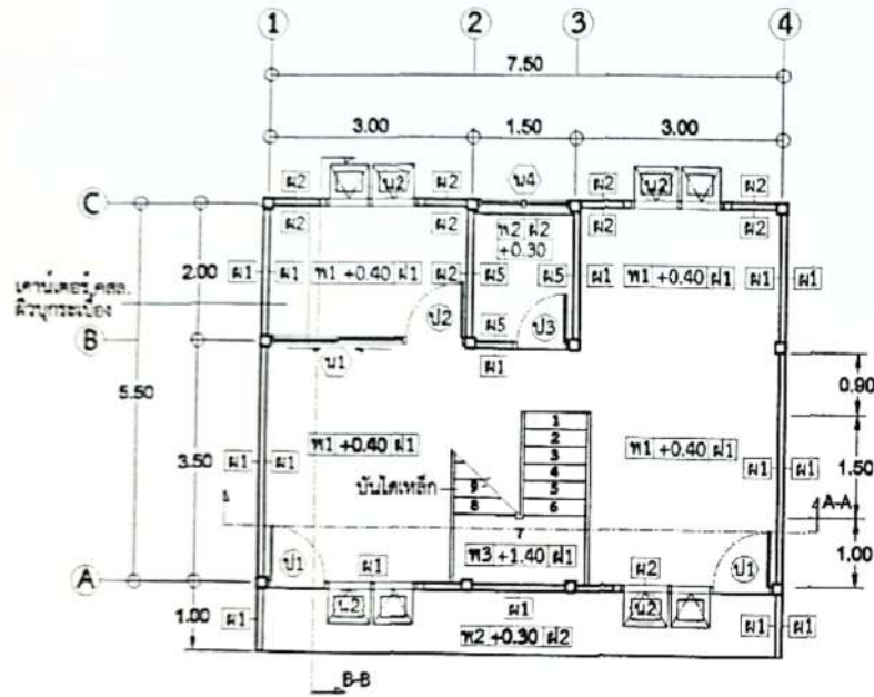
แบบพื้นชั้นล่าง SCALE 1:100
