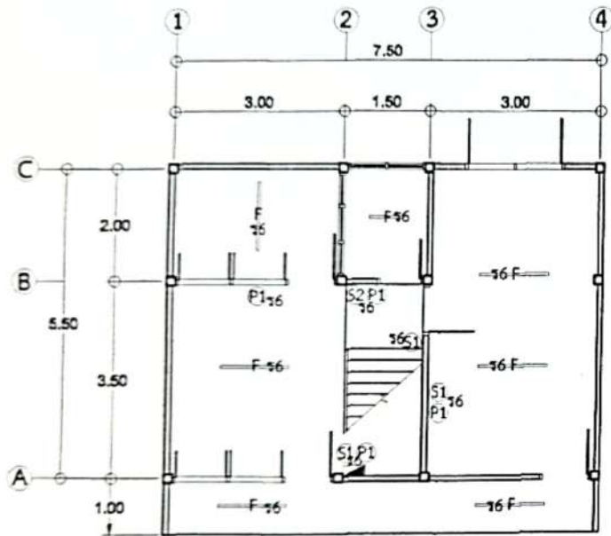
แบบไฟฟ้าชั้นล่าง (แบบเดิม) SCALE 1:100
