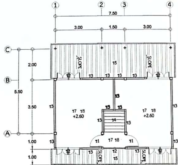
แบบพื้นชั้นบน (แบบเดิม)
