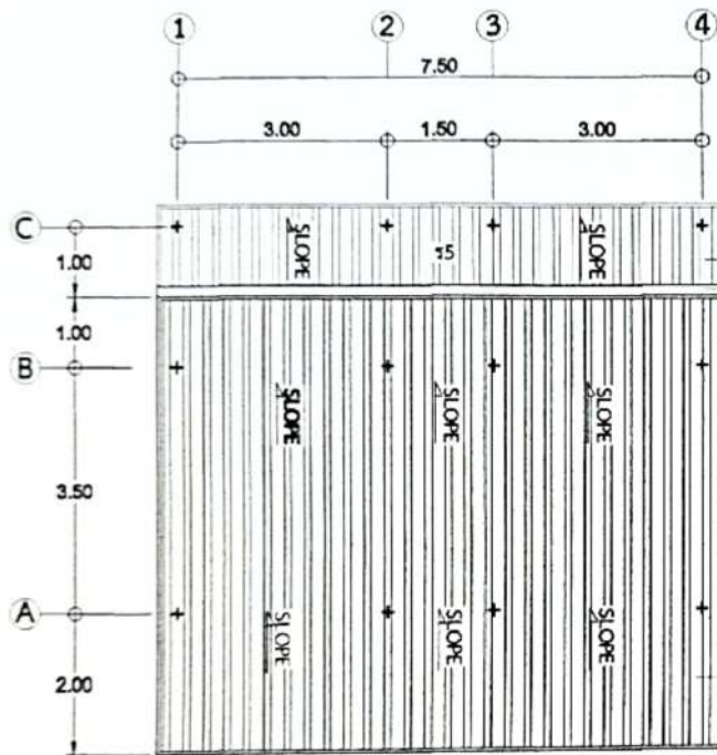
แบบหลังคา SCALE 1:100
