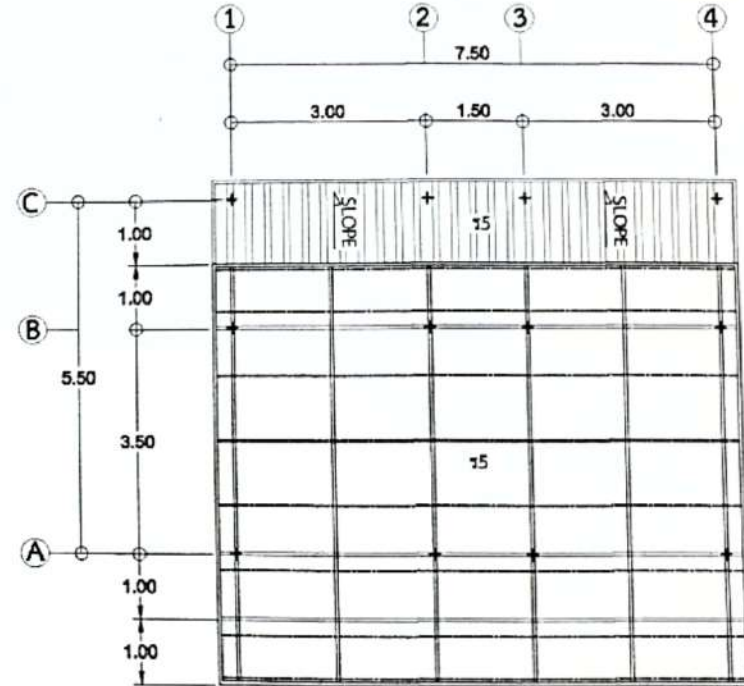
แบบโครงหลังคา (แบบเต็ม) SCALE 1:100
