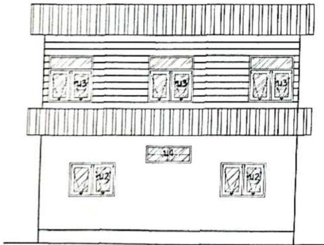
รูปด้าน ③ SCALE 1:100
