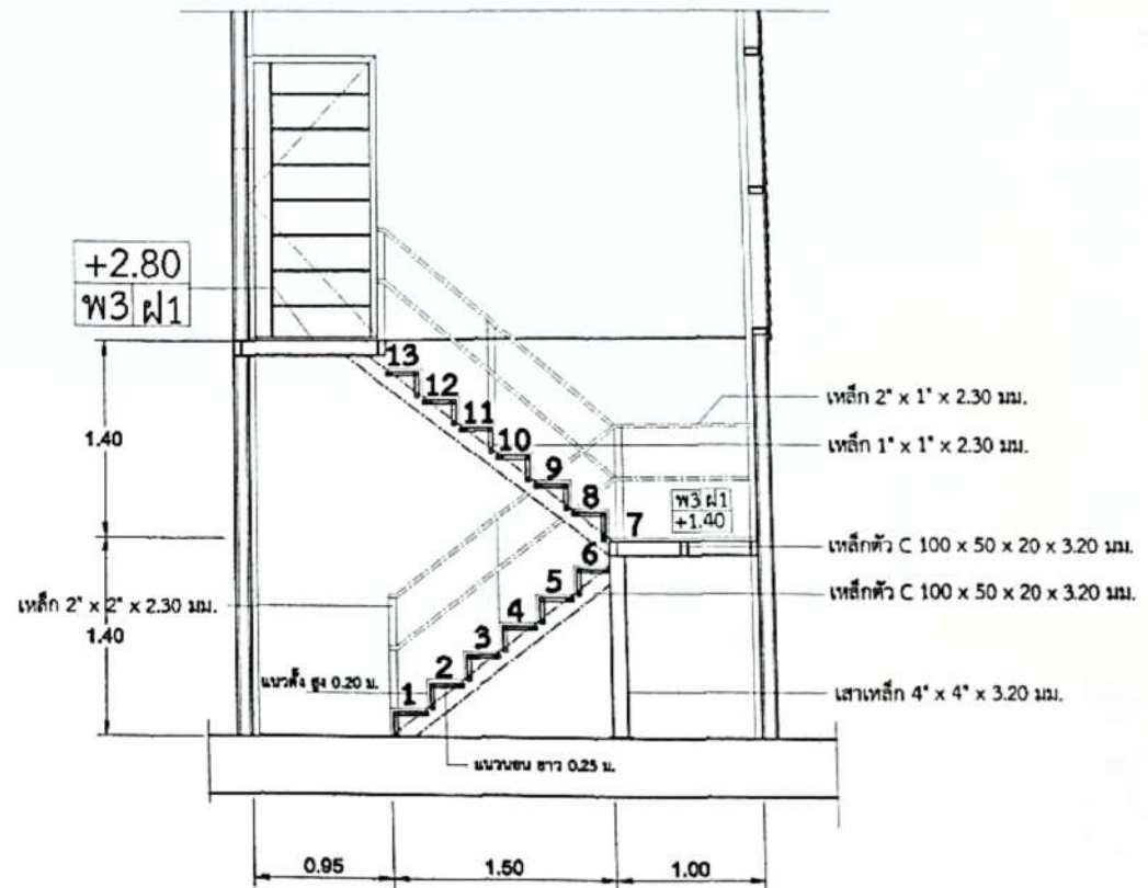
รูปตัดบันได SCALE 1:50
