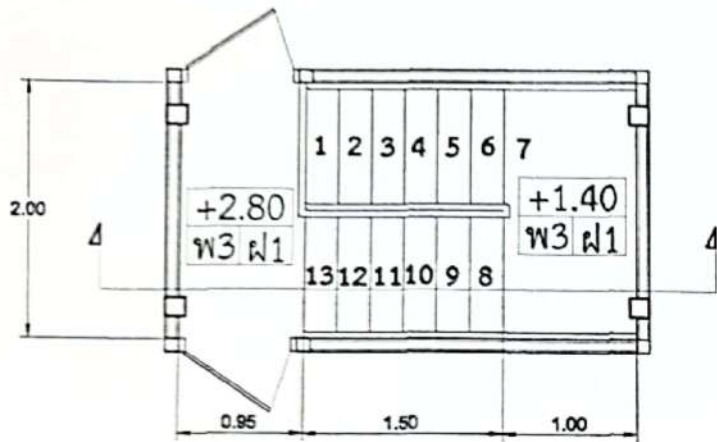
แบบขยายบันได SCALE 1:50
