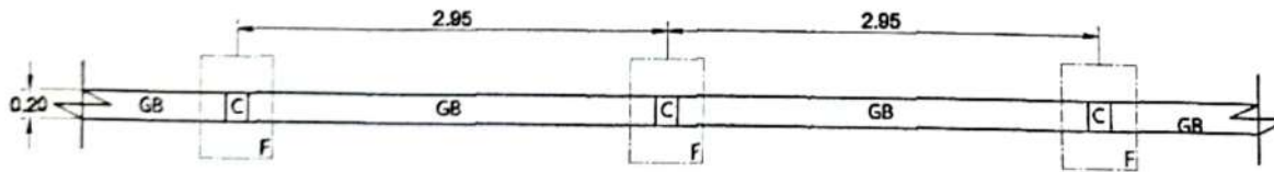
แบบฐานราก, คาน SCALE 1:50
