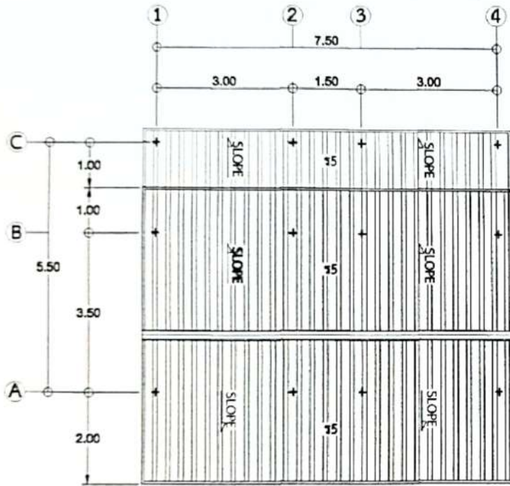
แบบหลังคา (แบบเต็ม) SCALE 1:100
