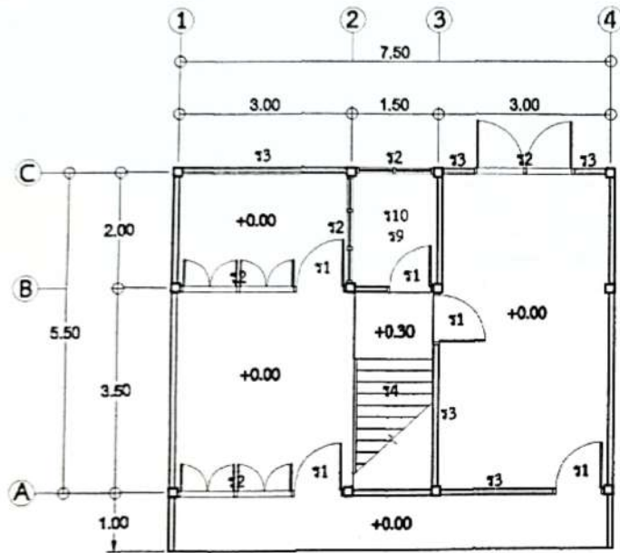
แบบพื้นชั้นล่าง (แบบเดิม)
