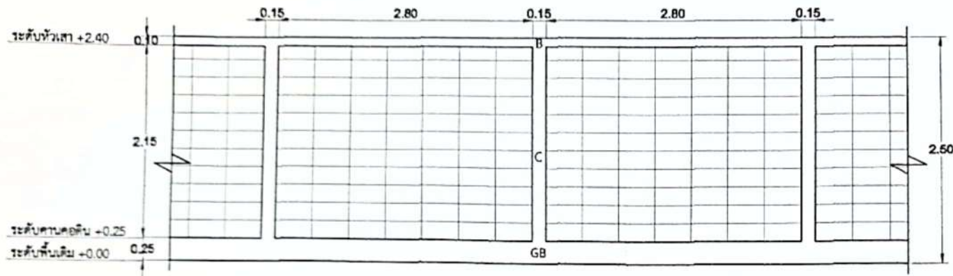
รูปด้าน SCALE 1:50
