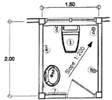
แบบขยายห้องน้ำ SCALE 1: 50
