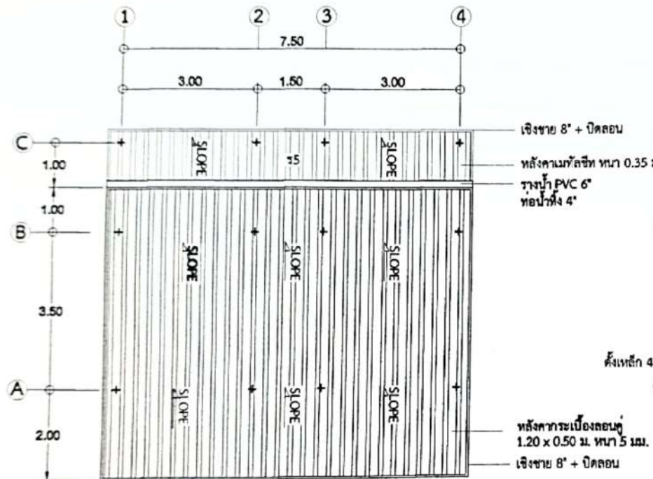
แบบหลังคา SCALE 1:100
