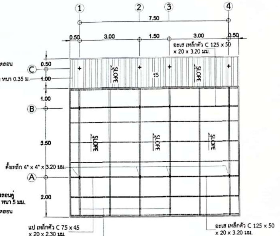
แบบโครงหลังคา SCALE 1:100
