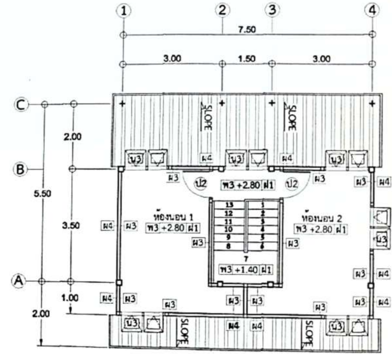
แบบพื้นชั้นบน SCALE 1:100
