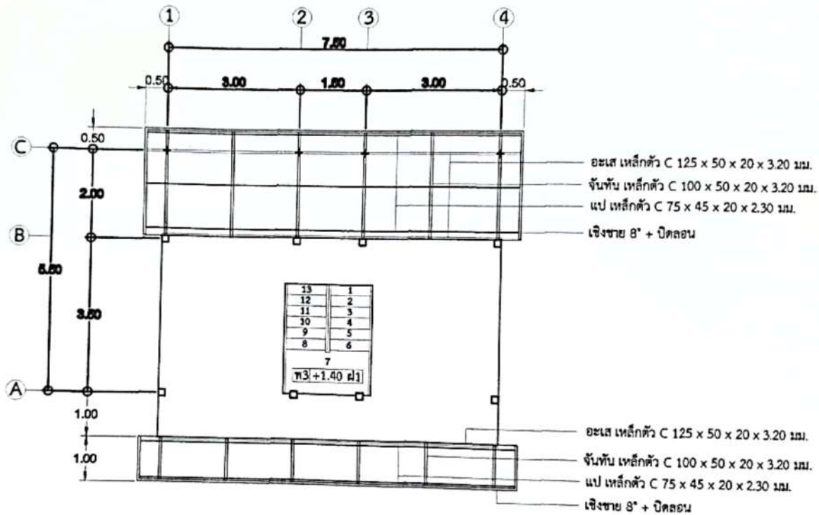
แบบโครงหลังคา (ห้องครัว, ด้านหน้า) SCALE 1:100
